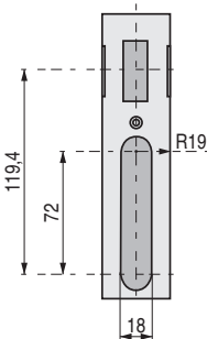
Detalle regulación del picaporte y cajetín de protección
